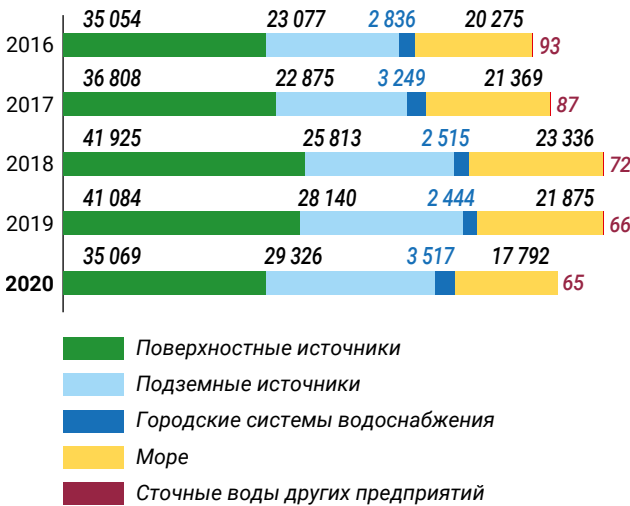
ВОДОЗАБОР ПО ГРУППЕ КОМПАНИЙ КМГ В РАЗБИВКЕ ПО ИСТОЧНИКАМ, 85 769 ТЫС. М³
